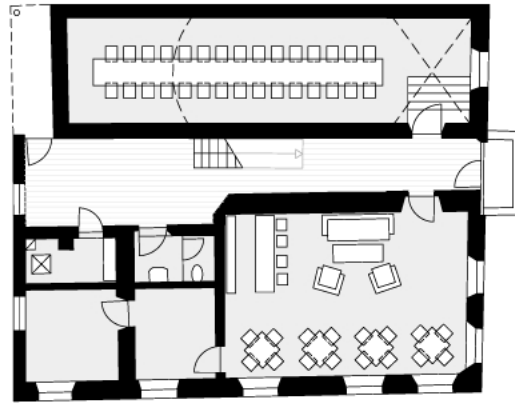
ERDGESCHOSS kommunale Nutzung
