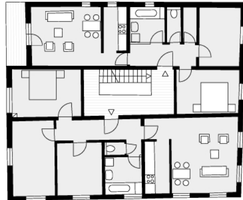
1. und 2. OBERGESCHOSS Wohnungen
